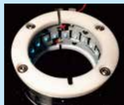
紫外線発光ダイオード(UV-LED)を用いたリングモジュール水消毒装置(特許第6208563号)
