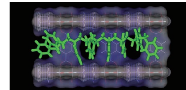
■ナノ空間に拘束された単分子鎖状のポリスチレン Single-stranded polystyrene constrained in the nanochannel.
