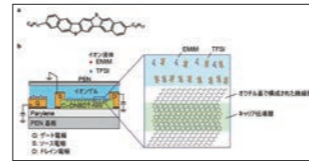
●図5 C8-DNBDTの単結晶を用いた電気二重層トランジスタ(EDLT)の概略図(左)とイオン液体とC8-DNBDTの界面の模式図(右)
