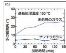
●図6 高温(150°C)処理後の水の接触角の時間依存性
