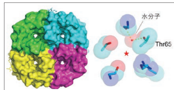
●図3 イネの生育に欠かせないケイ酸を透過させるチャンネルタンパク質の分子構造
