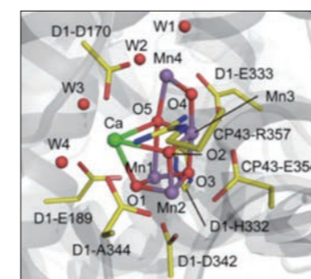
■光化学系II蛋白質に埋め込まれている水分解酸素発生触媒サイト \text{Mn}_4\text{CaO}_5 錯体 \text{Mn}_4\text{CaO}_5 cluster, the water-oxidation / \text{O}_2 -evolving site in Photosystem II
