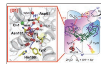
■ \text{Mn}_4\text{CaO}_5 錯体近傍の水分子からプロトンを引き抜き水分解反応を促進させるために必要な「蛋白質内プロトン移動経路」(左)と「長距離電子移動経路」(右) Proton transfer(left) and electron transfer pathways (right) required for water oxidation ( 2\text{H}_2\text{O} \rightarrow \text{O}_2 + 2\text{H}^+ + 4\text{e}^- ) in the \text{Mn}_4\text{CaO}_5 moiety of Photosystem II.
